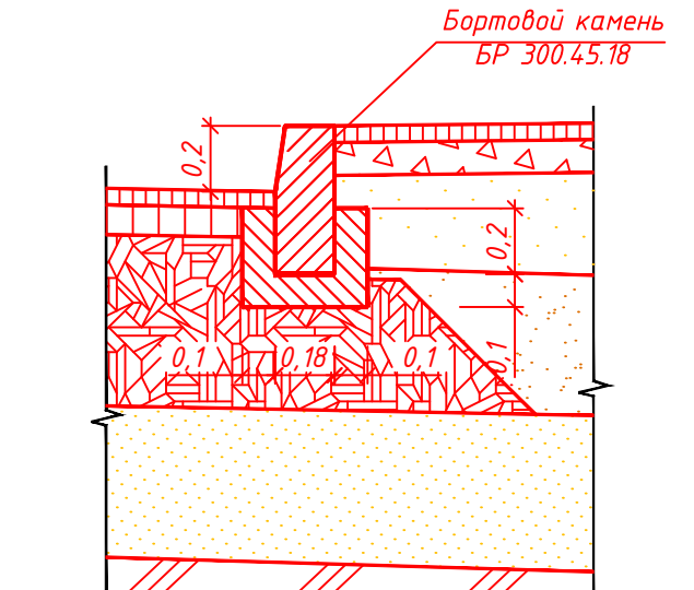
Узел А
